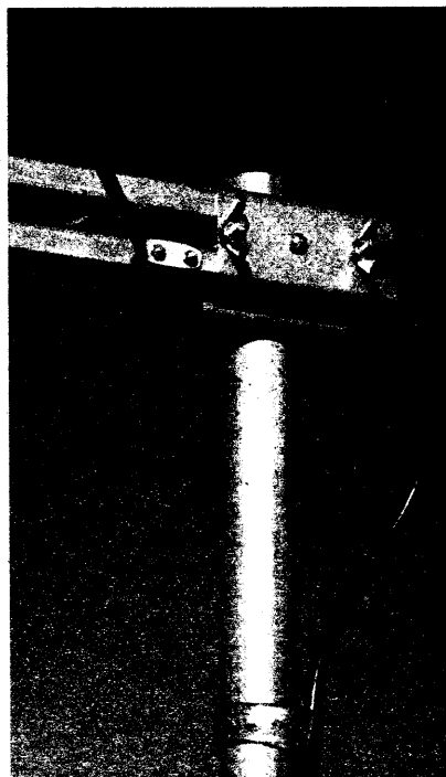
Obr. 9. Anténa se vzadu upevňuje přičtyčkou, která současně stabilizuje rozteč obou nosníků ráhna
